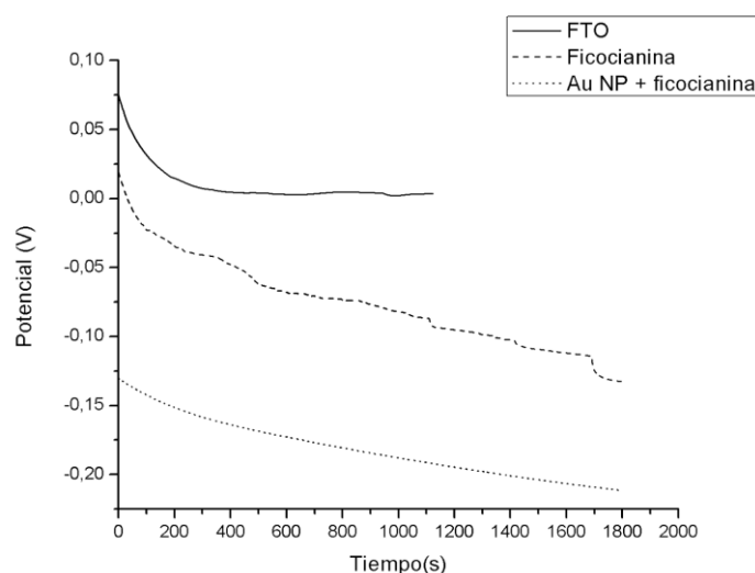
Figura 1. Potencial a circuito abierto en función del tiempo. En línea continua para el electrodo de FTO, en línea discontinua para el electrodo de FTO con ficocianina y en línea punteada el electrodo de FTO con nanopartículas de oro y ficocianina.
