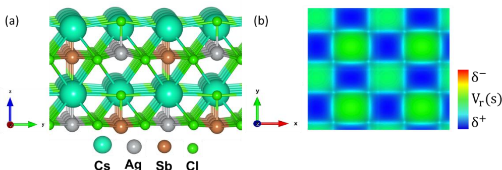
Figura 1: (a) Mapa morfológico e (b) de isosuperfície de potencial eletrostático.
